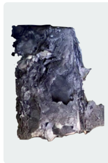
Batteria di terze parti dopo un test di sovraccarico abusivo, che ha lo scopo di simulare la ricarica della batteria oltre i limiti previsti.
